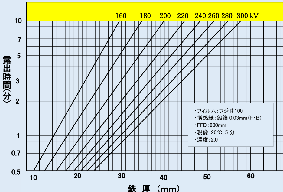
RIX-300MC-2 参考露出線図
