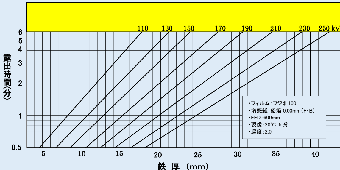
RIX-250C-2 参考露出線図
