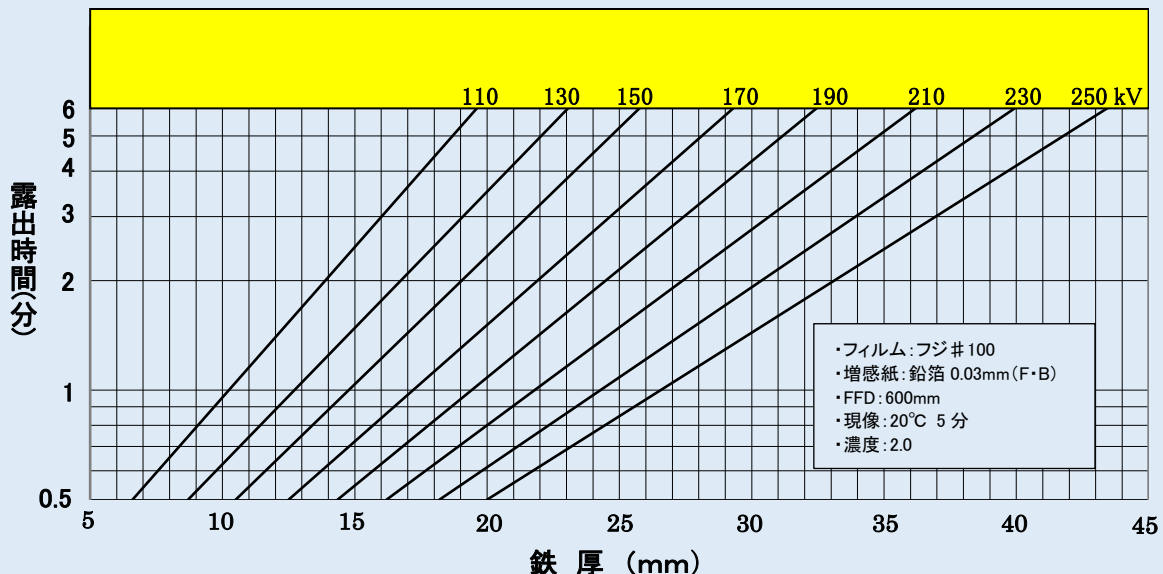
RIX-250C-2 参考露出線図
