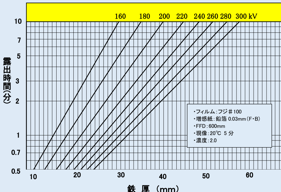
RIX-300MC-2 参考露出線図
